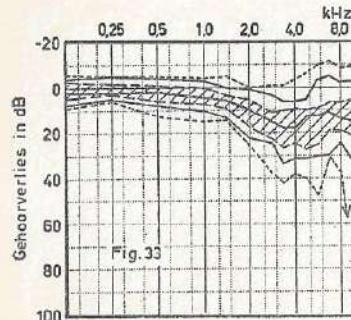
FIGUUR 33 - Constructiefabriek, lichtmetaal-afdeling (tijdens het werk; 22 uren).
