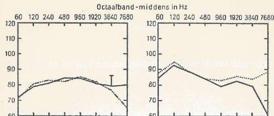
FIGUUR 9 - (getrokken) Automaten- afdeling; (gestippeld) Ponsery.
