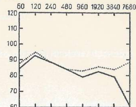
FIGUUR 10 - Aluminium spuitgiets- afdeling. (getrokken) algemeen niveau, compressoren; (gestippeld) ontsnap- pende perslucht.
