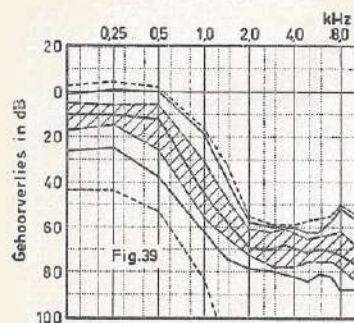
FIGUUR 39 - Scheepswerf, kokers (tijdens het werk; 20 oren).
