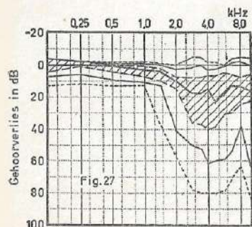
FIGUUR 27 - Dynamoblikponserij (vóór het werk; 32 uren).
