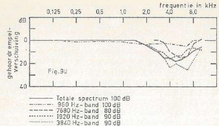
FIGUUR 90 - De tijdelijke gehoordrempelverandering door inwerking gedurende 5 minuten van het lawaai van dribbelbanen in een chocoladefabriek, resp. van de afzonderlijke octaafband-componenten daarvan op hetzelfde sterkteniveau als waarin ze in het totale spectrum gemeten zijn.
