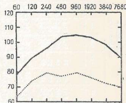
FIGUUR 6 - Zware plaatwerkerij. (getrokken) op het bordes; (gestippeld) algemeen niveau zonder lawaaig werk.
