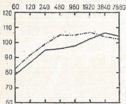
FIGUUR 5 - Zware plaatwerkerij. (getrokken) een hakker; (gebroken) twee hakkers.
