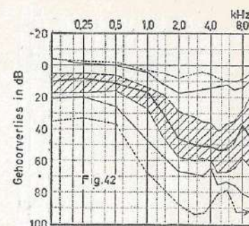
FIGUUR 42 - Scheepswerf, klinkerhulpen (tijdens het werk; 26 oren).
