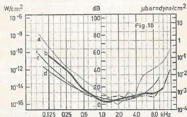
FIGUUR 18 - De gebruikte nulcurve voor het onderzoek van elk oor afzonderlijk met een telefoon.
