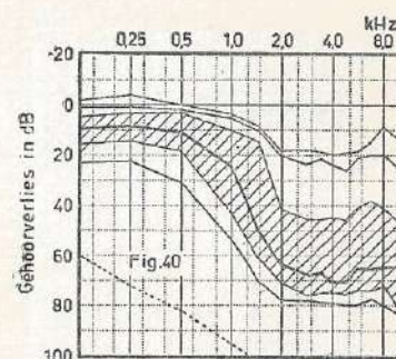
FIGUUR 40 - Scheepswerf, klinkers (tijdens het werk; 24 oren).
