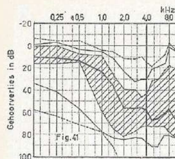
FIGUUR 41 - Scheepswerf, aanhouders (tijdens het werk; 18 oren).
