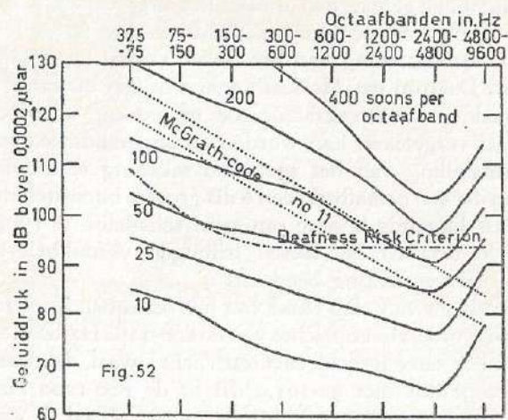
FIGUUR 52 - Vergelijkend overzicht van de classificaties van lawaai in verband met de invloed op het optreden van beroepshardhorendheid.
