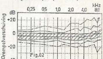
FIGUUR 82 - Ponseriej.
