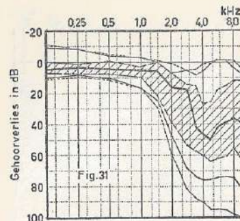
FIGUUR 31 - Constructiefabriek, zware plaatwerkerij (tijdens het werk; 16 uren).
