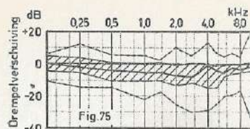
FIGUUR 75 - Praletta-afdeling, arbeiders met 3 maanden of meer expositietijd (22 uren).
