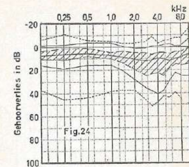
FIGUUR 24 - Chocoladefabriek, Praletta-afdeling (vóór het werk; 40 oren).
