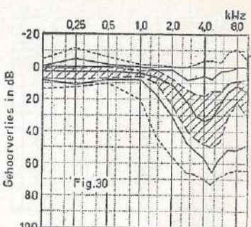
FIGUUR 30 - Constructiefabriek, ketelmakers (tijdens het werk; 38 uren).
