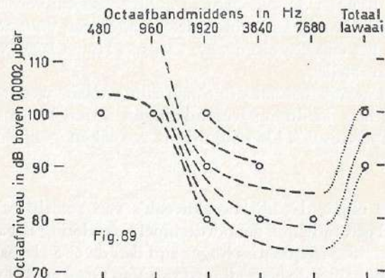
FIGUUR 89 - „Isotraumatische lijnen”. Met deze lijnen is weergegeven bij welke niveau's de verschillende octaafbandruisen een even grote maximale drempelverschuiving gaven bij expositie gedurende 5 minuten.
