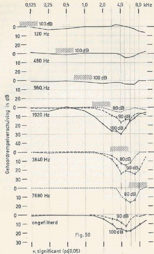
FIGUUR 50 - Drempelverschuiving door expositie gedurende 5 minuten aan verschillende componenten van fabriekslawaai [4 proefpersonen].
