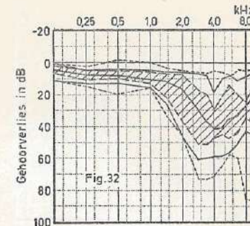
FIGUUR 32 - Constructiefabriek, draaijerij (tijdens het werk; 14 uren).
