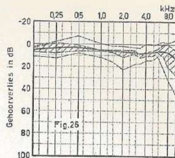
FIGUUR 26 - Biscuitbakkerij (tijdens het werk; 10 uren).
