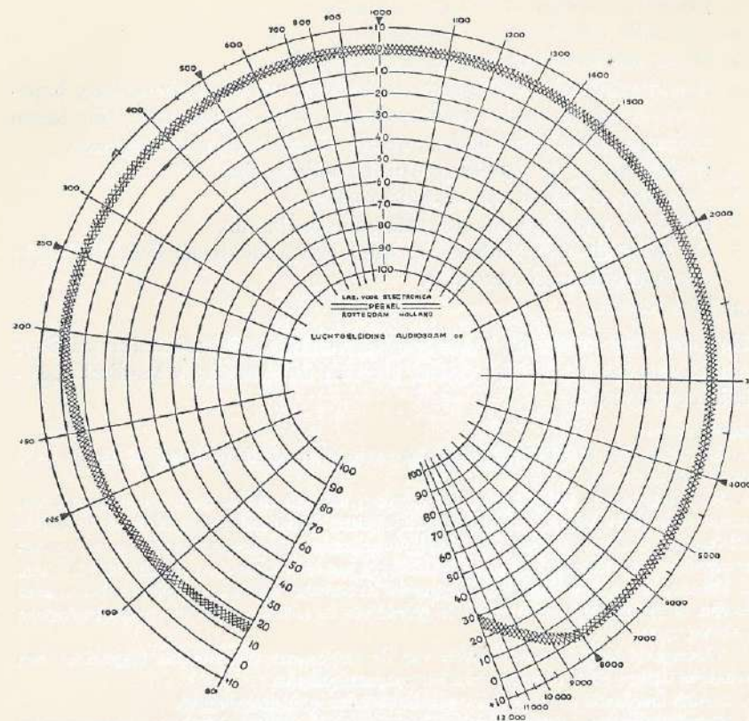
FIGUUR 15 - Voorzijde van de audiogramkaart (luchtgeleiding) van de Van Dishoeck-audiometer, fabriek Peekel
