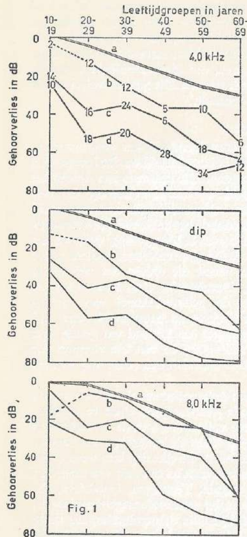
FIGUUR 1 - De invloed van de leeftijd op de gehoordrempel van arbeiders in fabriekslawaai.
