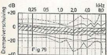
FIGUUR 79 - Praletta- en Lehmann-Savy-afdeling, arbeiders met 3 maanden of meer expositietijd (30 uren).
