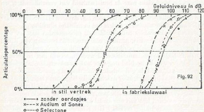
FIGUUR 92 - Spraakaudiogrammen, opgenomen terwijl de uitwendige gehoorgang al of niet afgesloten was met een gehoorbeschermers van een type, dat geheel afsluit [Audium of Sonex] of van een type, dat de lage tonen ongehinderd laat passeren [Selectone].
