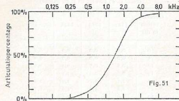
FIGUUR 51 - Het verband tussen het articulatiepercentage voor lettergrepen en de bovengrens van het doorlaat-gebied van een filter, dat van de aangeboden spraak de lage tonen wel, maar de hoge niet doorlaat. Men ziet dat, wanneer de tonen boven 1500 Hz uit de aangeboden spraak weggenomen zijn, de lettergreep-verstaanbaarheid toch nog 50% bedraagt, wat volgens tabel 7 een zinnen-verstaanbaarheid van 96% meebrengt. [Ontleend aan Kryter, naar gegevens van French & Steinberg]
