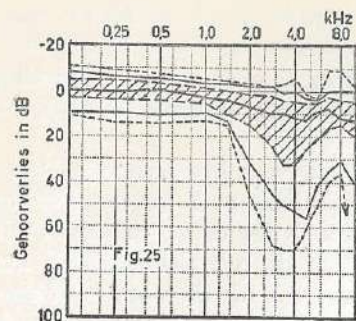
FIGUUR 25 - Chocoladefabriek, Lehmann-Savy-afdeling (vóór het werk; 24 uren).
