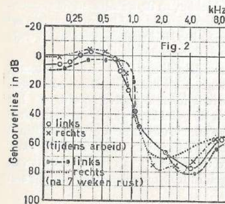
FIGUUR 2 - Audiogram van een 30-jarige man, die 6 jaar als constructieklinker werkt. Een gewoon gesprek met de onderzoeker kan steeds zonder merkbare moeite verstaan worden.
