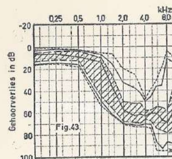
FIGUUR 43 - Scheepswerf, boorders (tijdens het werk; 10 oren).
