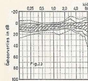
FIGUUR 23 - Chocoladefabriek, enrobeuse-afdeling (tijdens het werk; 42 oren).
