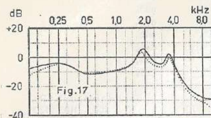
FIGUUR 17 - Frequentiekaracteristiek van de bij het onderzoek te Dordrecht gebruikte telefoons (links en rechts).
