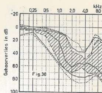
FIGUUR 38 - Scheepswerf, ketelmakers (tijdens het werk; 14 oren).
