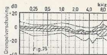
FIGUUR 76 - Praletta-afdeling, arbeiders met minder dan 3 maanden expositietijd (10 uren).
