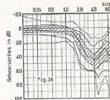
FIGUUR 36 - Constructiefabriek, plaat- drijvers (tijdens het werk; 20 uren).
