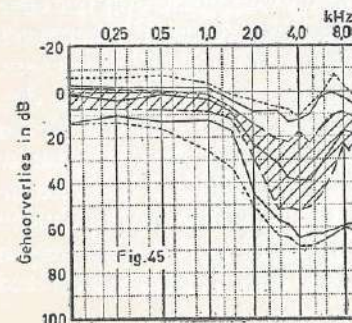
FIGUUR 45 - Scheepswerf, plaatwerkers (tijdens het werk; 20 oren).
