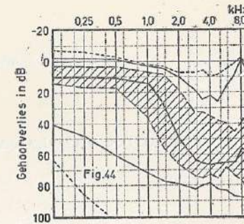
FIGUUR 44 - Scheepswerf, ijzerwerkers (tijdens het werk; 24 oren).
