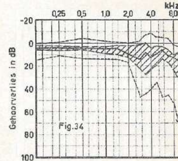
FIGUUR 34 - Constructiefabriek, gereedschapmakerij (tijdens het werk; 14 uren).
