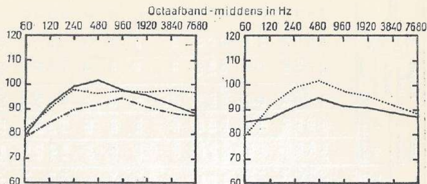
FIGUUR 3 - Chocoladefabriek. (getrokken) Lehmann-machine; (gestippeld) Lehmann- en Savy- machine; (gebroken) Praetta-machine.
