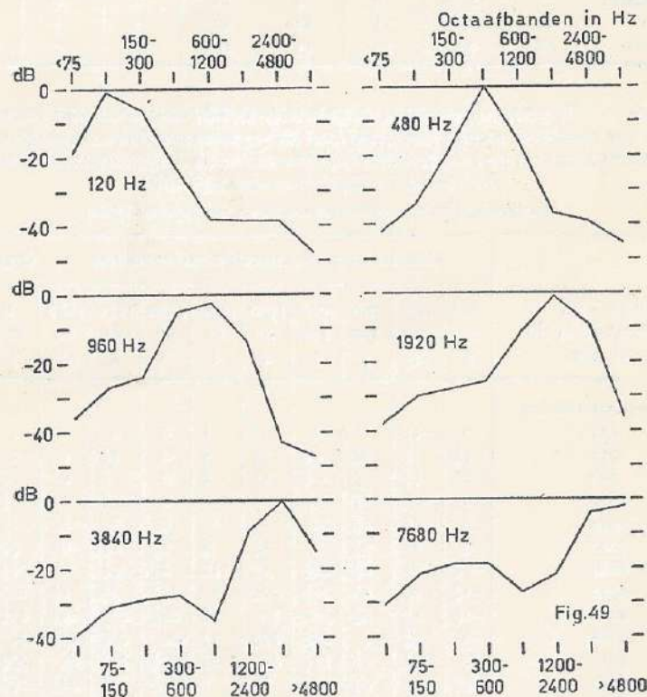
FIGUUR 49 - De spectra van het via octaafbandfilters opgenomen fabriekslawaai [intensiteitsverschillen in dB per octaaf ten opzichte van het totale niveau].
