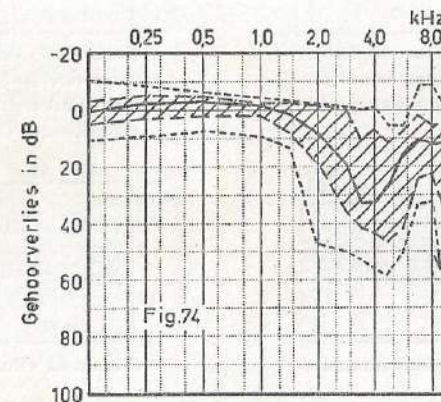
FIGUUR 74 - Lehmann-Savy-afdeling, arbeiders met 3 maanden of meer expositietijd, vóór het werk [8 oren].
