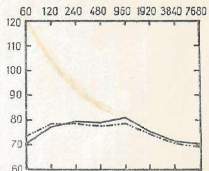
FIGUUR 8 - Sigarettenmachines. (getrokken) tussen de machines; (gebroken) bij bureau zaalcontroleuse
